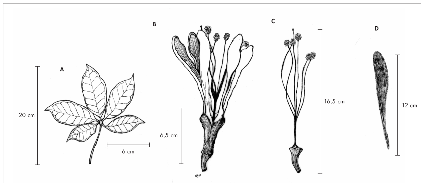
Fig. 2. – Ceiba samauma (Mart.) K. Schum. A. Hoja; B. Flor; C. Androecium; D. Detalle del indumento de la superficie exterior en un pétalo. [De Egea & al. 1203, FCQ] [Ilustrado por G. Colombino]
